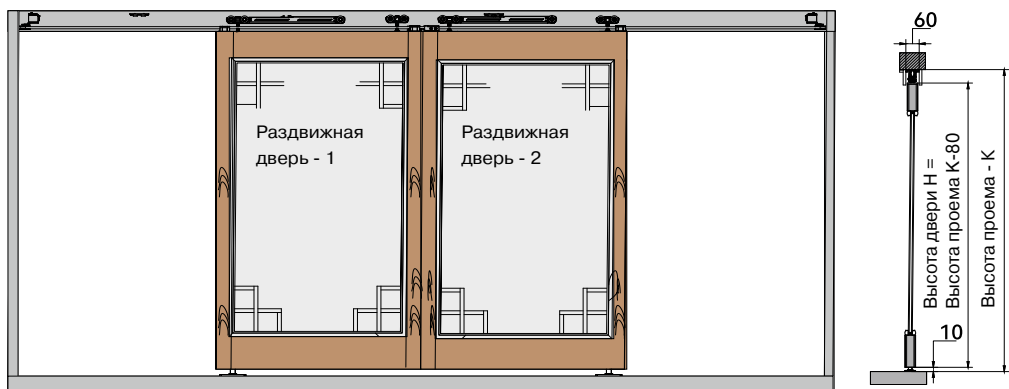
Расчет размера двери для системы FM911A
