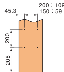
Схема присадки фасада при установке направляющих с правой стороны
