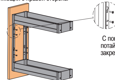
Схема присадки фасада при установке направляющих с правой стороны
