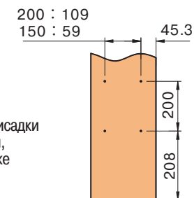
Схема присадки фасада при установке направляющих с левой стороны
